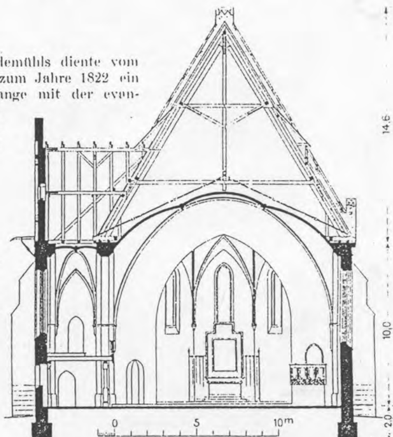
Abb. 2. Querschnitt.
