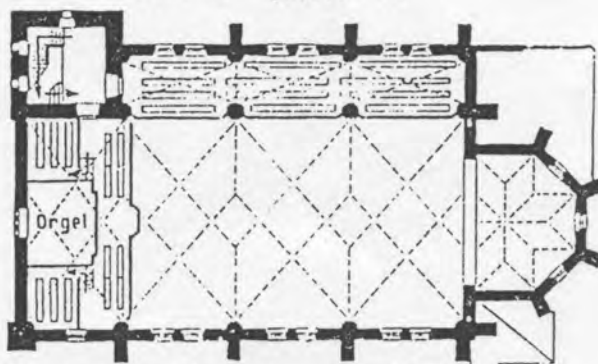
Abb. 4. Grundriß in Emporenhöhe.
