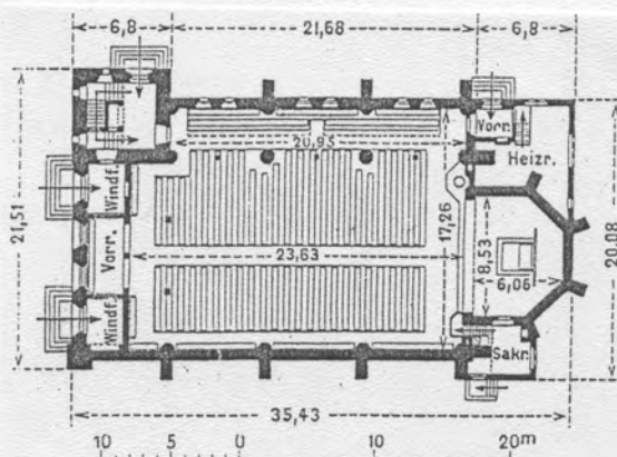
Abb. 5. Grundriß zu ebener Erde.
