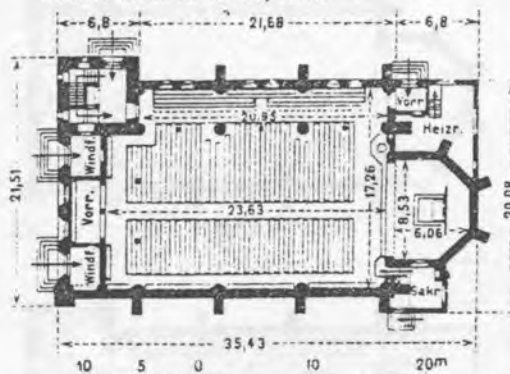
Abb. 5. Grundriß zu ebener Erde.
