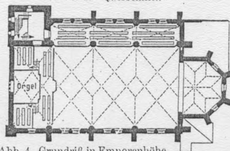
Abb. 4. Grundriß in Emporenhöhe.
