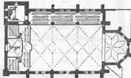
Abb. 4. Grundriß in Emporenhöhe.
