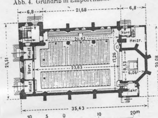
Abb. 5. Grundriß zu ebener Erde.
