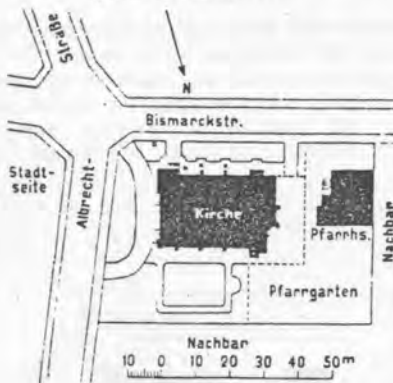
Abb. 1. Lageplan.
