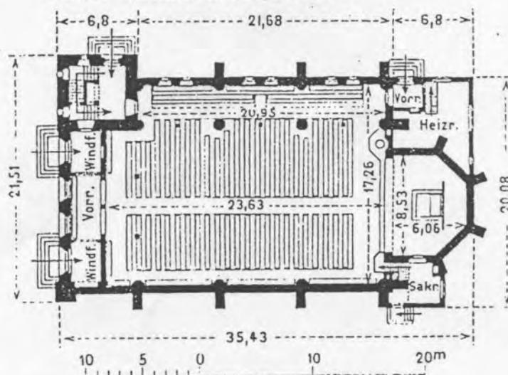
Abb. 5. Grundriß zu ebener Erde.
