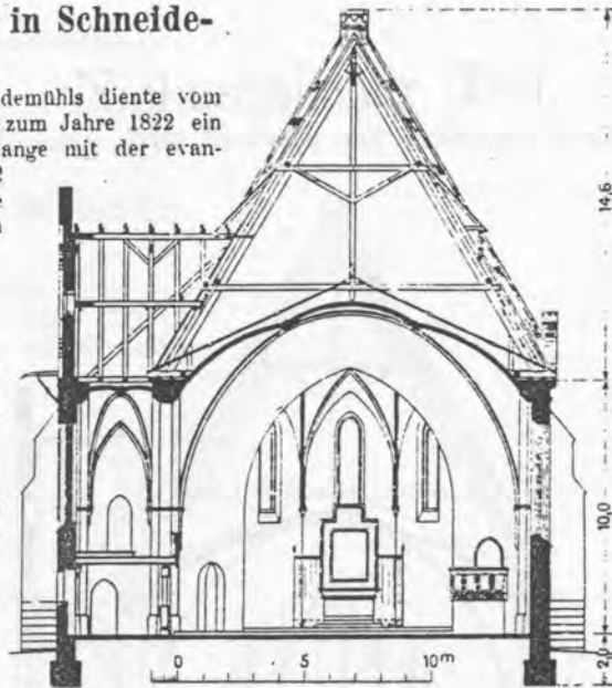
Abb. 2. Querschnitt.
